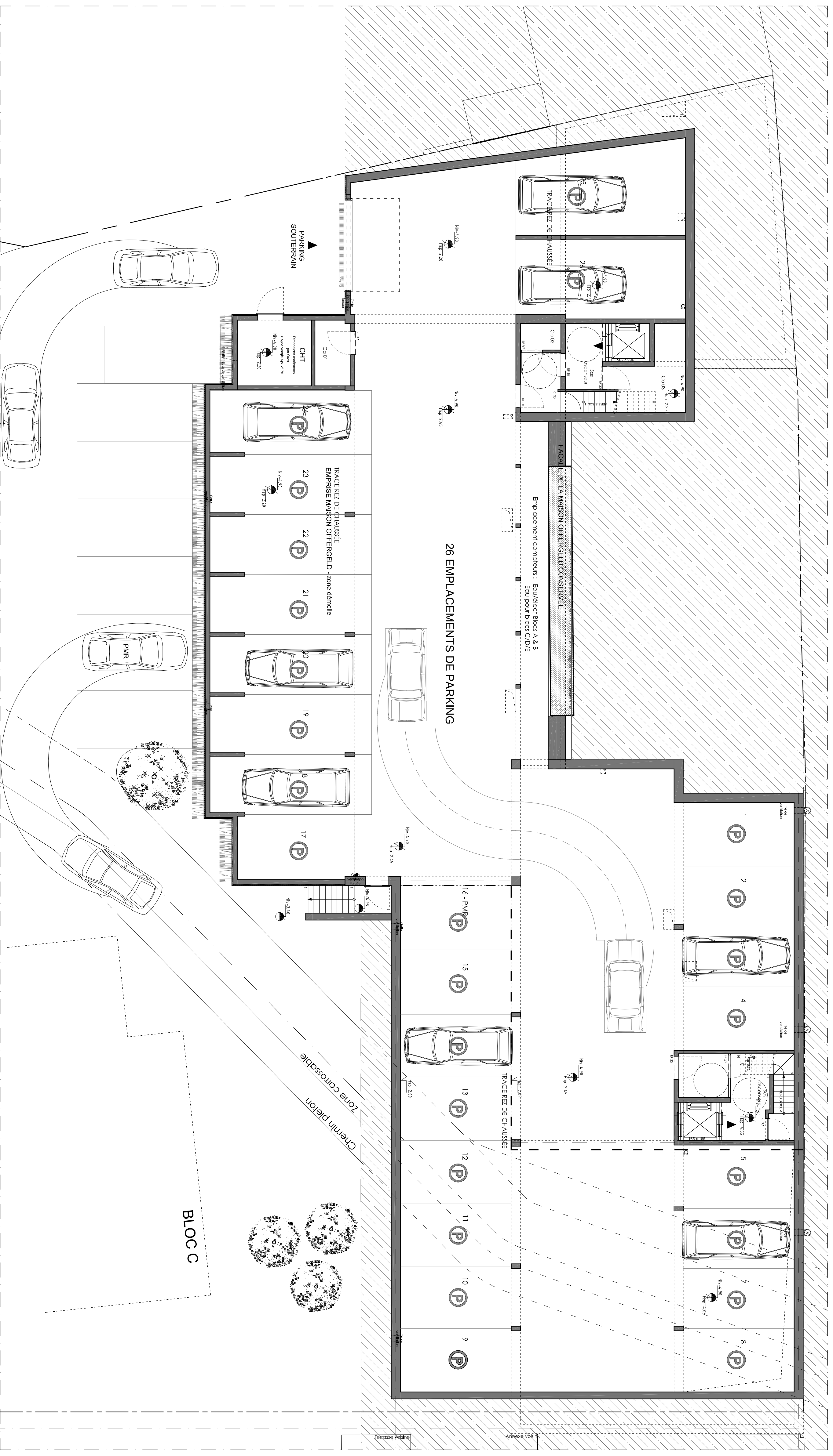
Plan sous-sol -2
